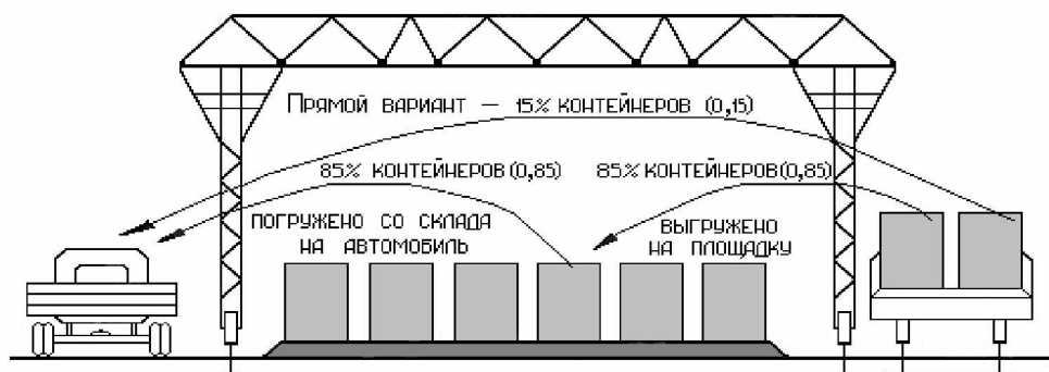
Рисунок 2 – Поясняющая схема к расчету среднесуточного объема грузопереработки
