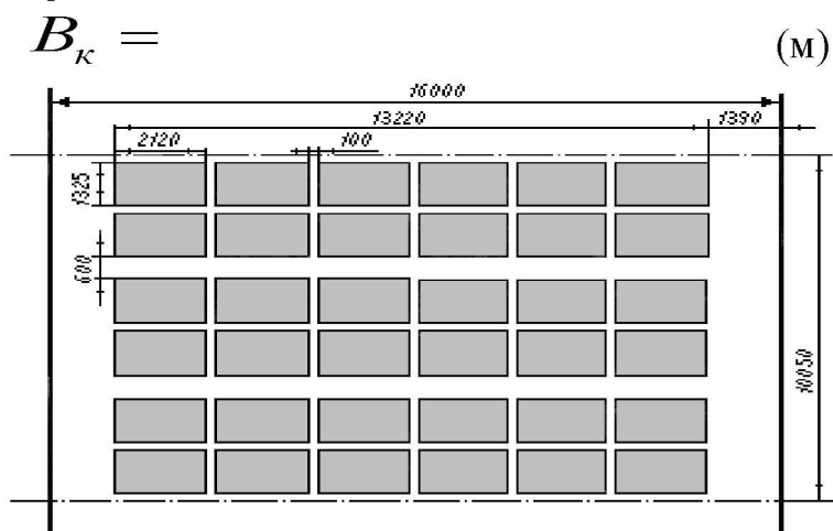
Рисунок 2 – Схема размещения контейнеров на площадке, обслуживаемой краном пролетом 16 м
