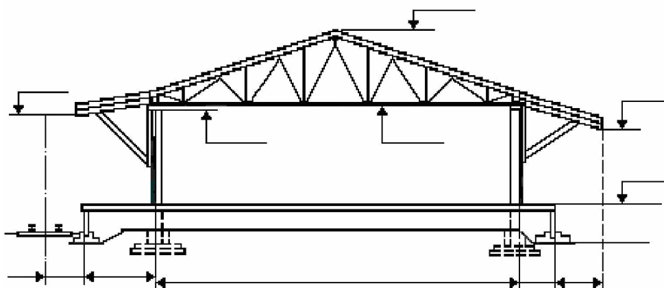
Рисунок 1 – Крытый прирельсовый склад для переработки тарно-упаковочных грузов
