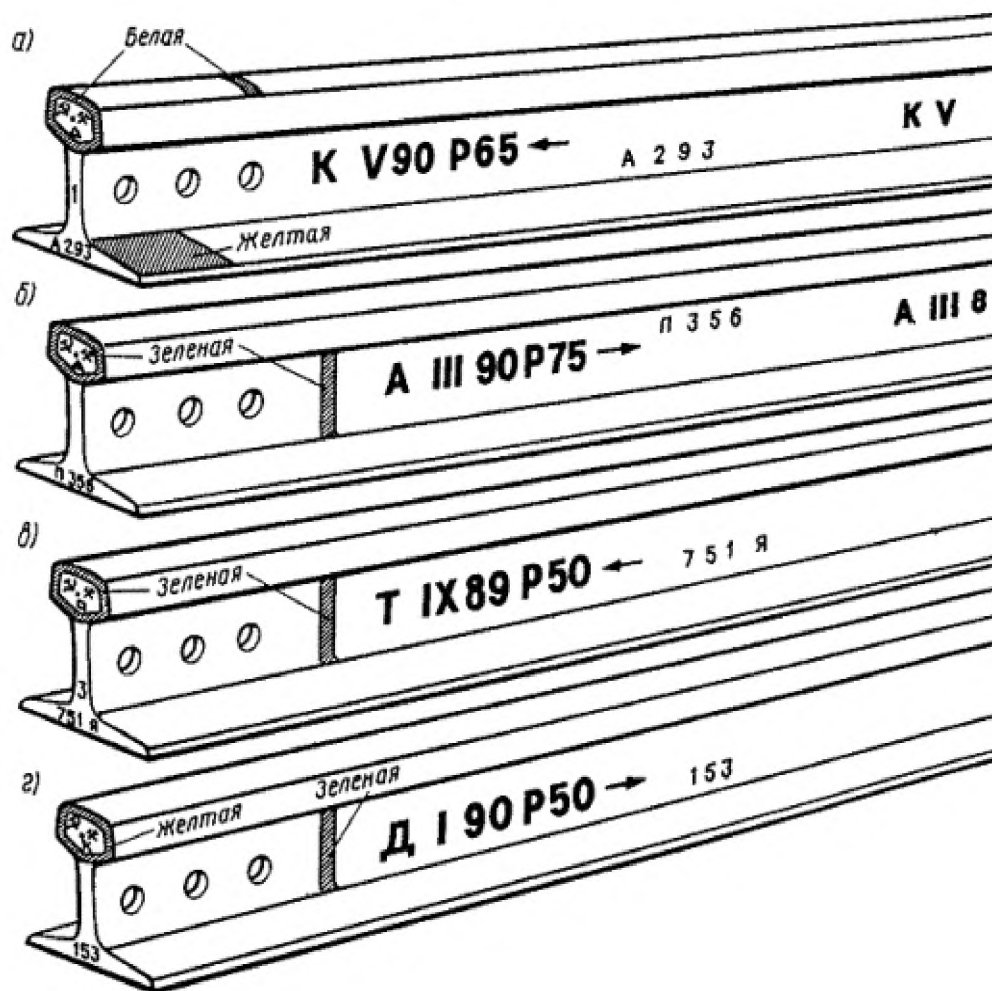
Рис. 4.1 Маркировка рельсов
