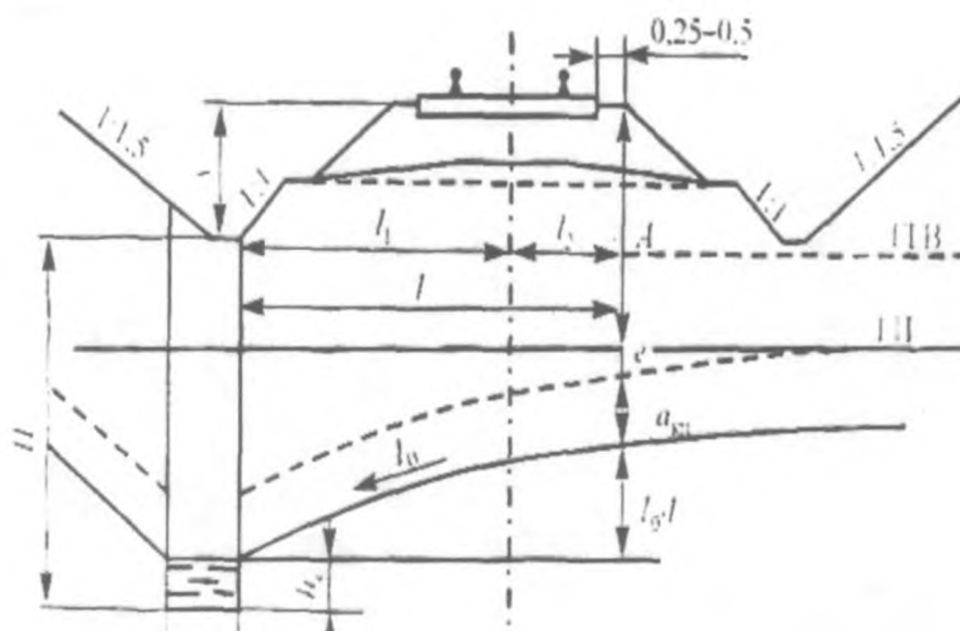
Рис. 3.1 Схема одностороннего подкюветного дренажа
