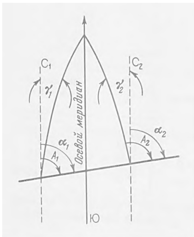
Рис. 2. Сближение меридианов
